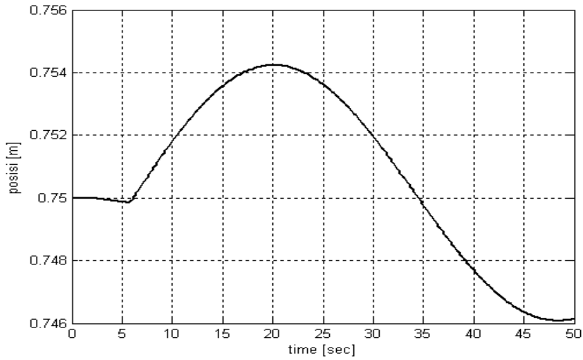
Posisi Pengendara terhadap ranah dengan sepeda motor dengan suspensi
