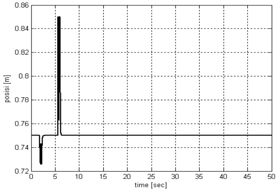
Posisi Pengendara terhadap ranah dengan sepeda motor tanpa suspensi
