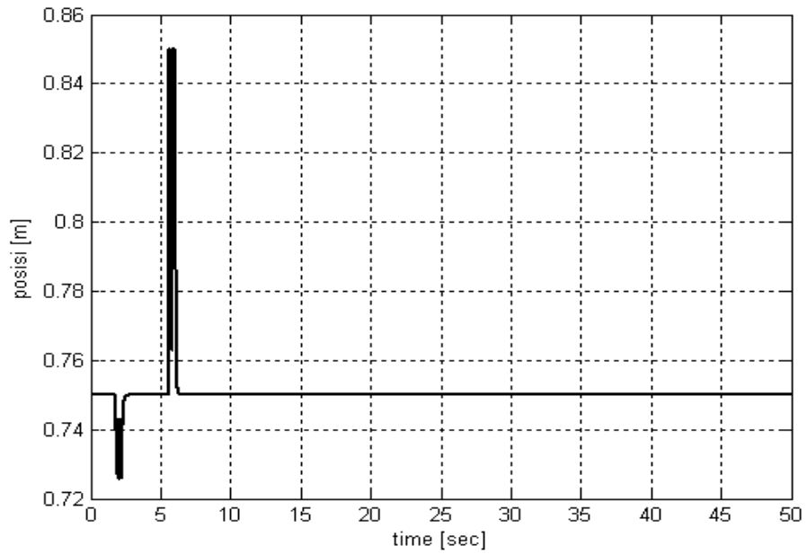
Posisi Pengendara terhadap ranah dengan sepeda motor tanpa suspensi
