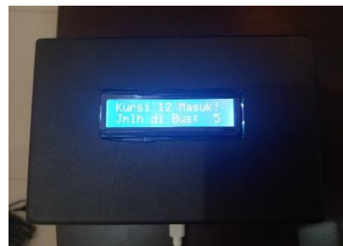
Gambar 18 Tampilan LCD Saat diberi Halangan Pada Sensor Masuk
