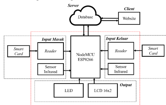
Gambar 1 Blok Diagram Rancangan Sistem
