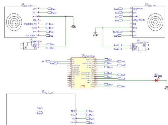
Gambar 2 Skematik Rancangan Perangkat Keras Alat Penghitung Penumpang
