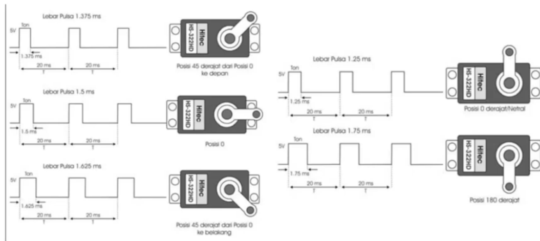
Gambar 3. 5 Prinsip Kerja Motor Servo
