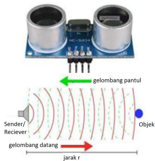
Gambar 2. 5 Sensor jarak ultrasonik dan prinsip kerjanya
