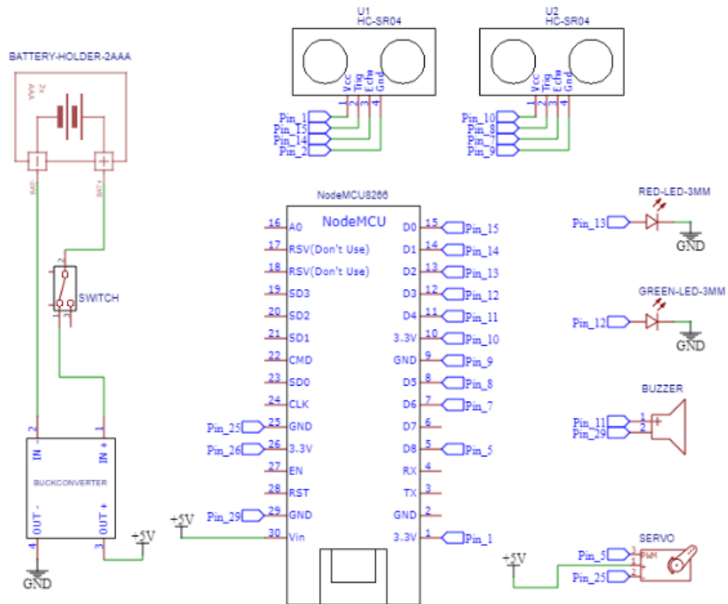
Gambar 3. 3 Skematik Rancangan Perangkat Keras Smart Trash
