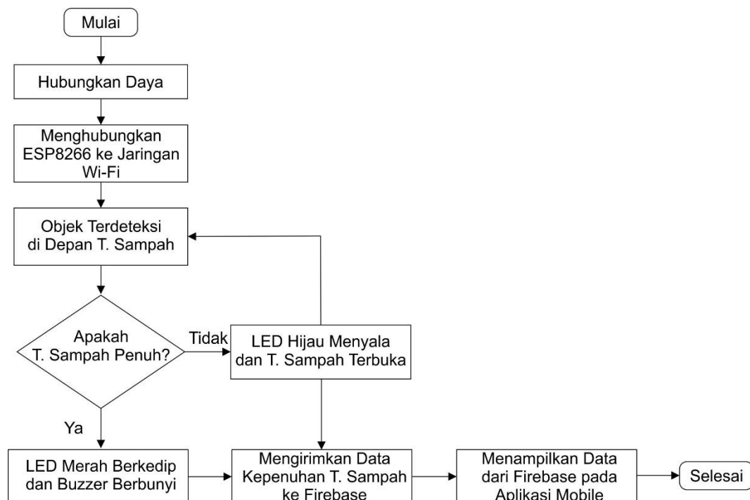
Gambar 3. 2 Flowchart Sistem Monitoring Smart Trash Pada Gedung Perkantoran Berbasis Android
