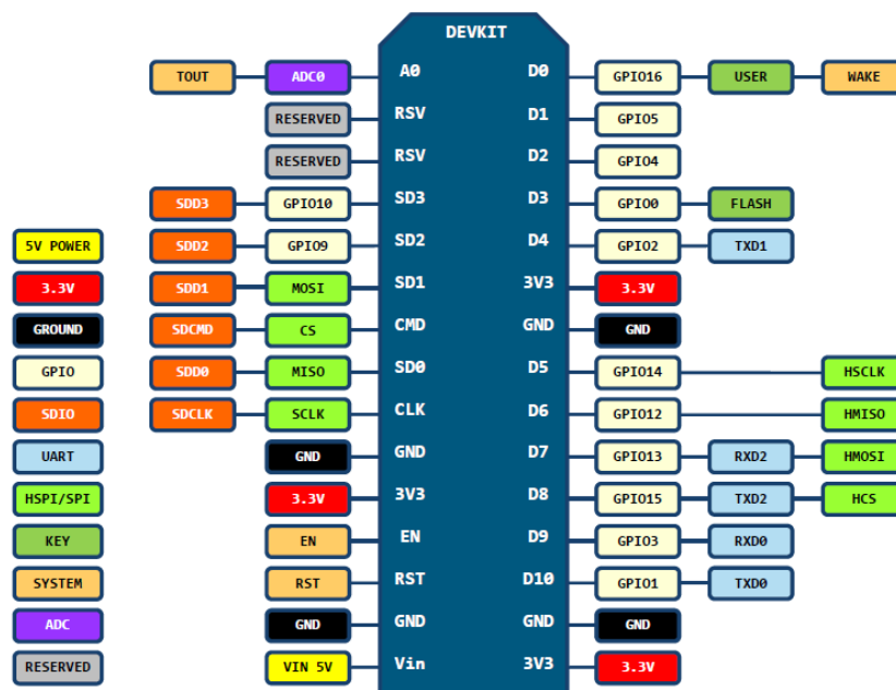
Gambar 2. 3 Konfigurasi pin NodeMCU
