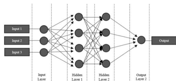
Gambar 2. MLP dengan 2 hidden layer
