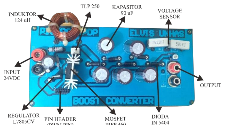
Gambar. 4. Tampilan Fisik Multilevel Boost Converter
