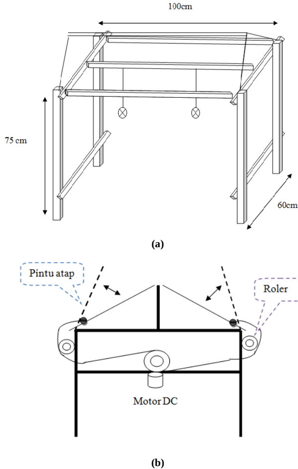
Gambar 8(a) Prototipe Sistem 8(b) Rancangan motor untuk buka tutup atap
