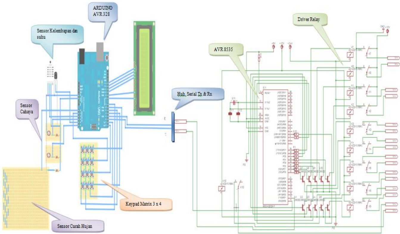
Gbr 4. Rangkaian Hardware elektronik
