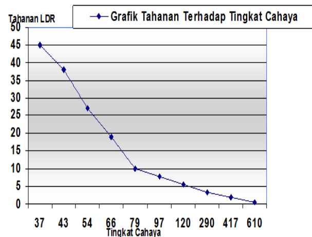
Gambar 6. Grafik tahanan LDR terhadap tingkat cahaya
