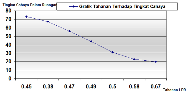
Gambar 10. Grafik tahanan LDR terhadap tingkat cahaya pada uji kecerahan rumah kaca
