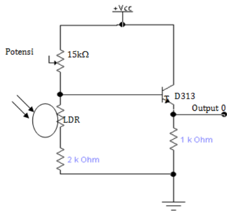
Gambar 5. Sensor LDR pada saat output logika 0
